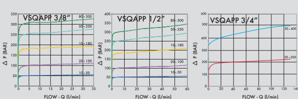
PRESSIONE/PORTATA PRESSURE/FLOW
