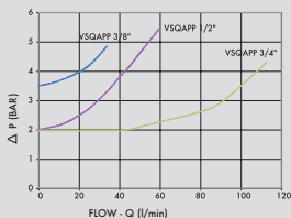
PERDITE DI CARICO PRESSURE DROP CURVE
